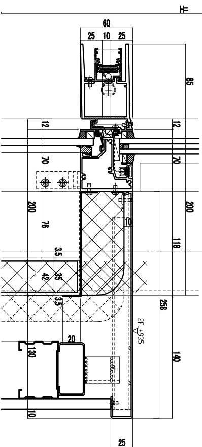
縦断面図
