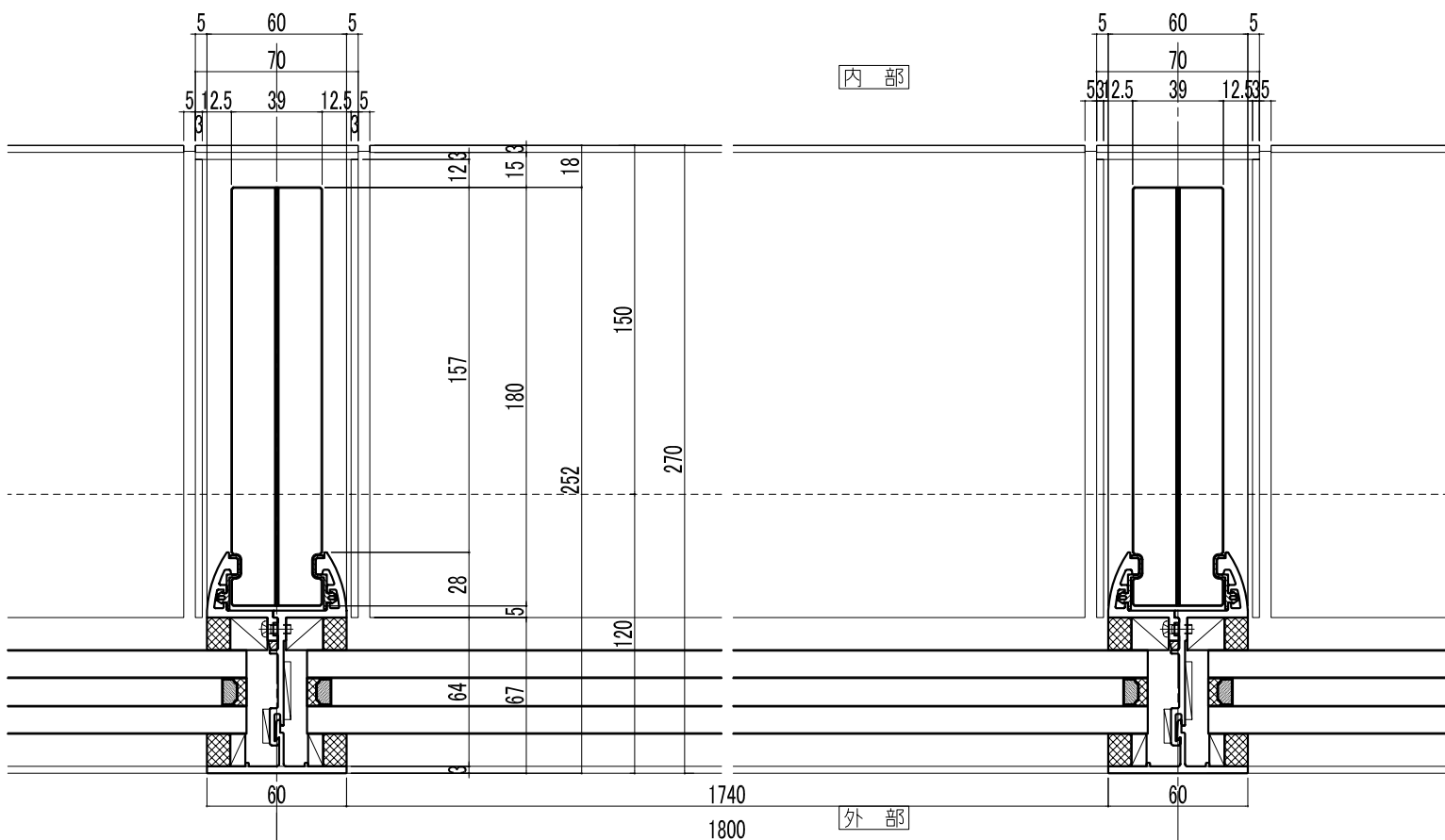
横断図
