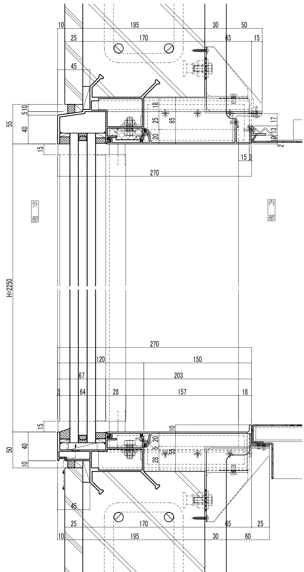
縦断図
