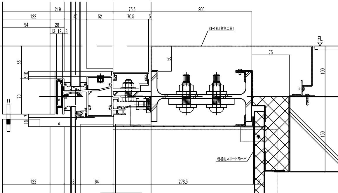
縦断図
