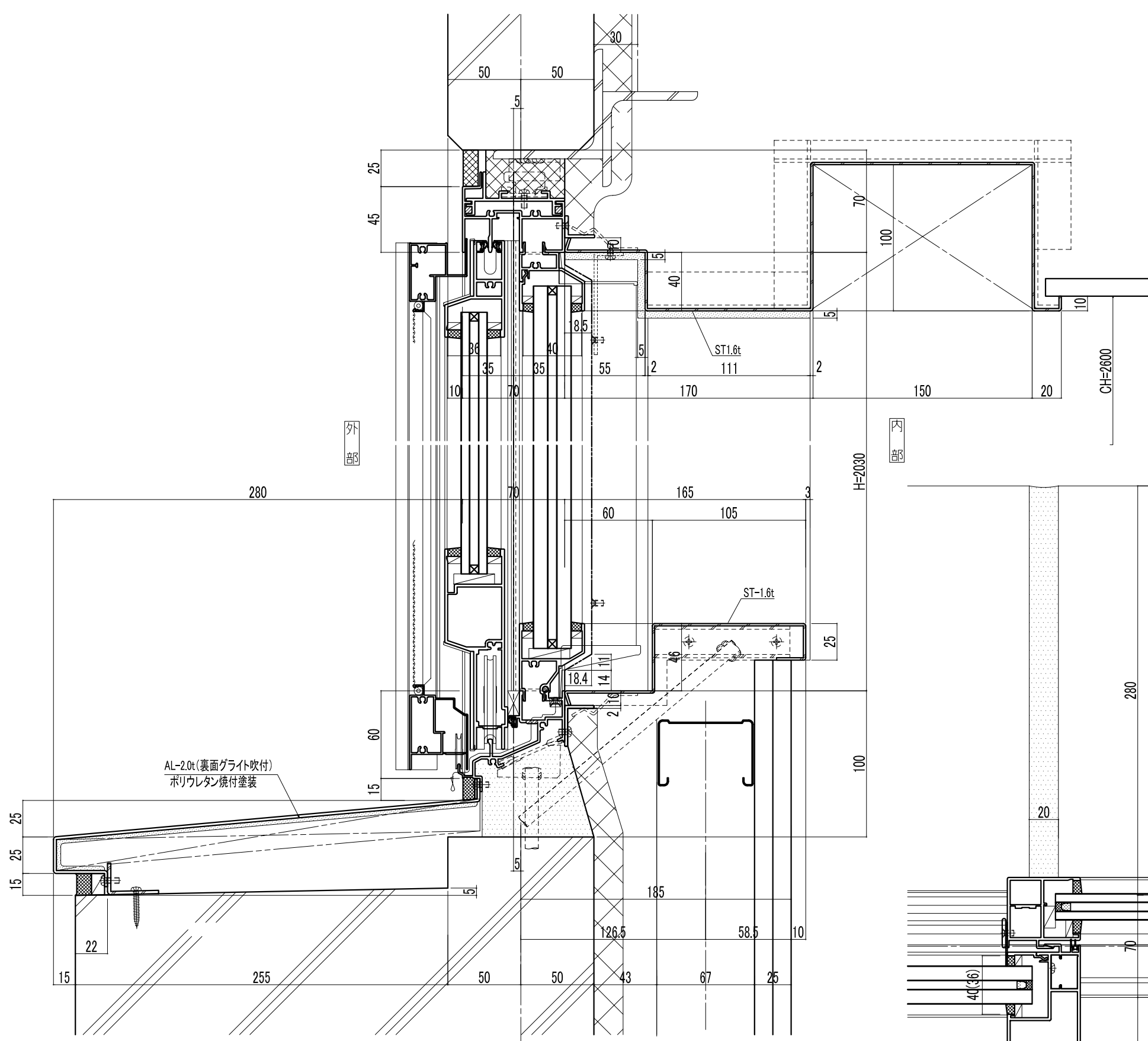
縦断図
