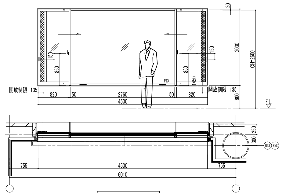
外観図
