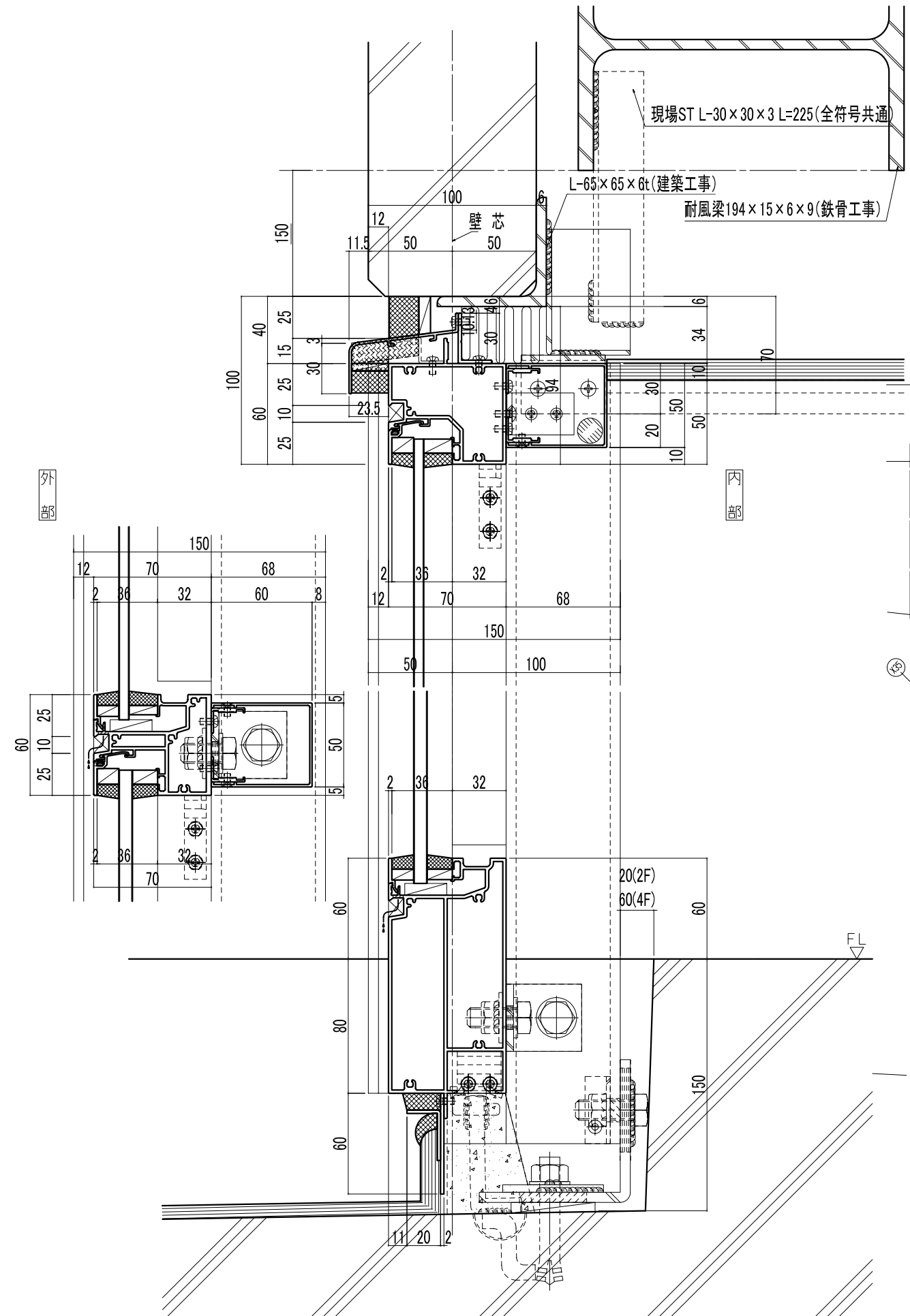
縦断図
