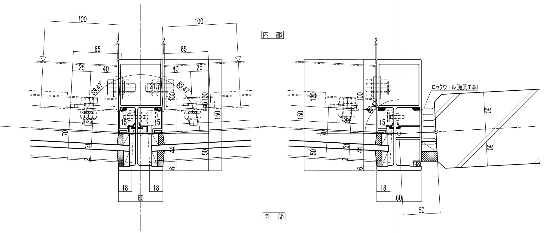
横断図
