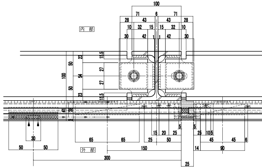
横断図
