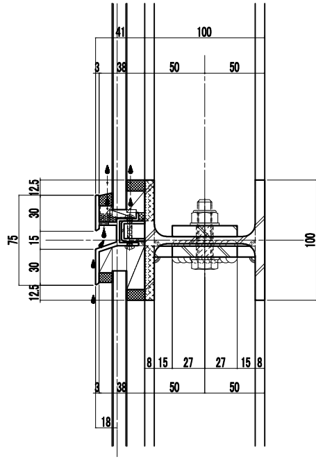
縦断図
