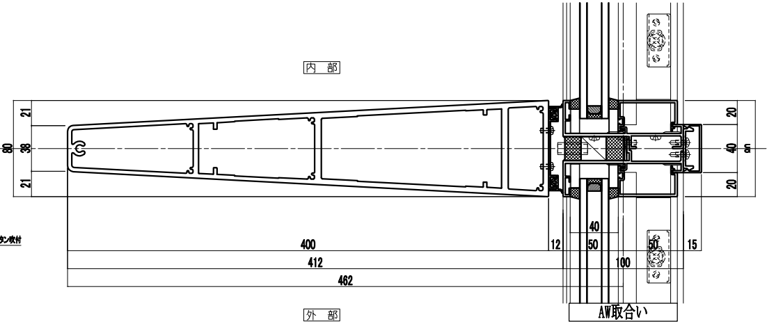
横断図
