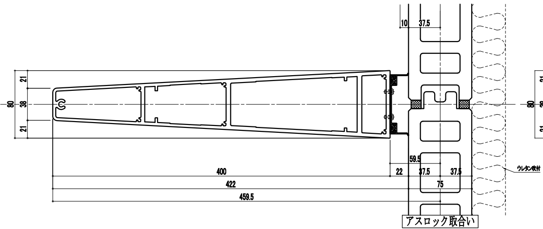
縦断図
