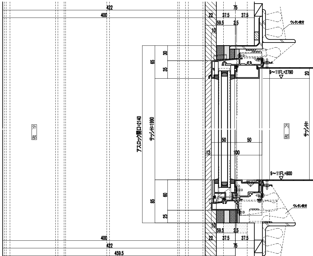
縦断図
