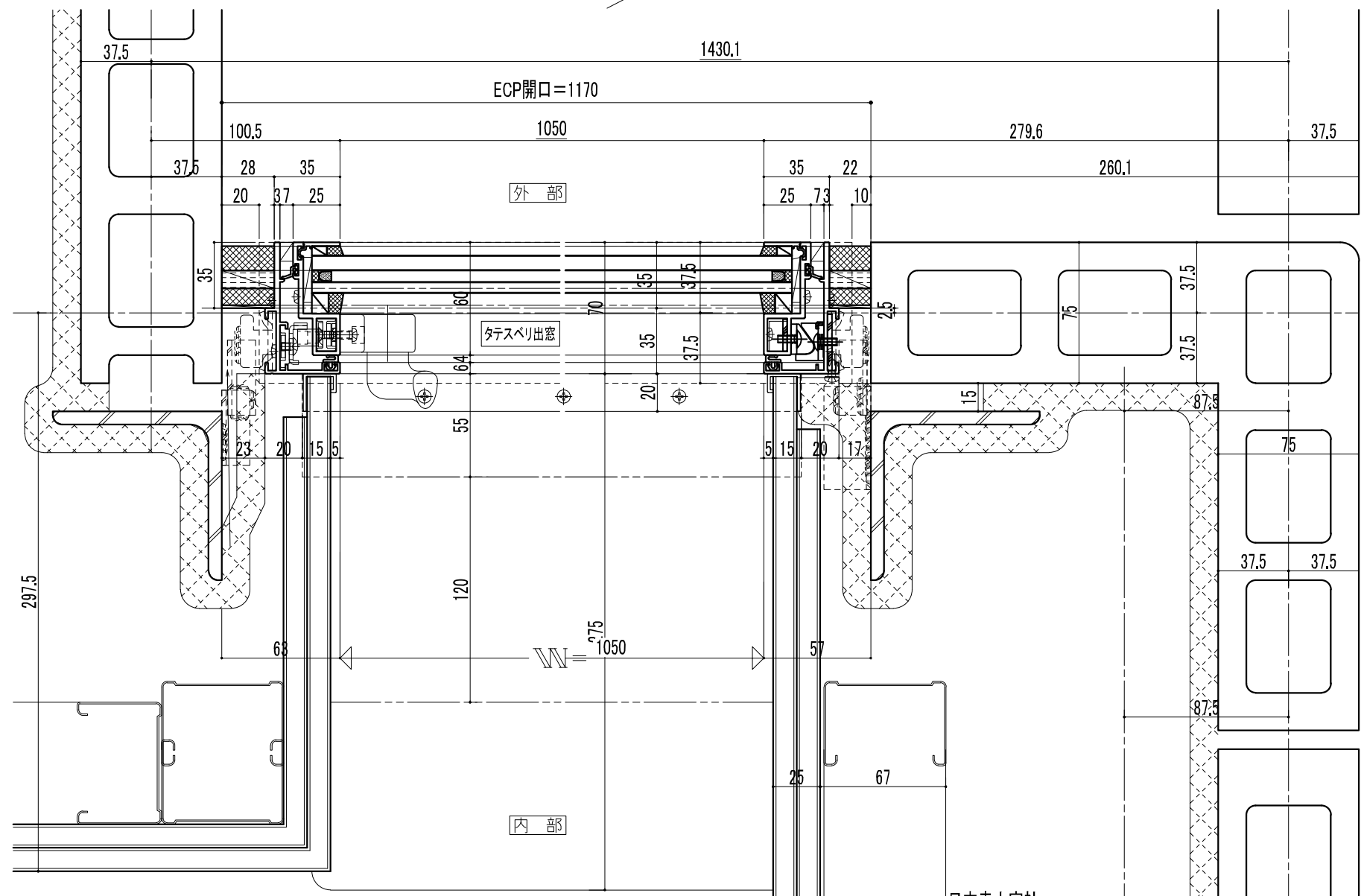
横断図
