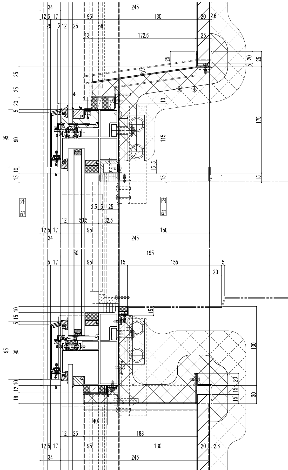
縦断図
