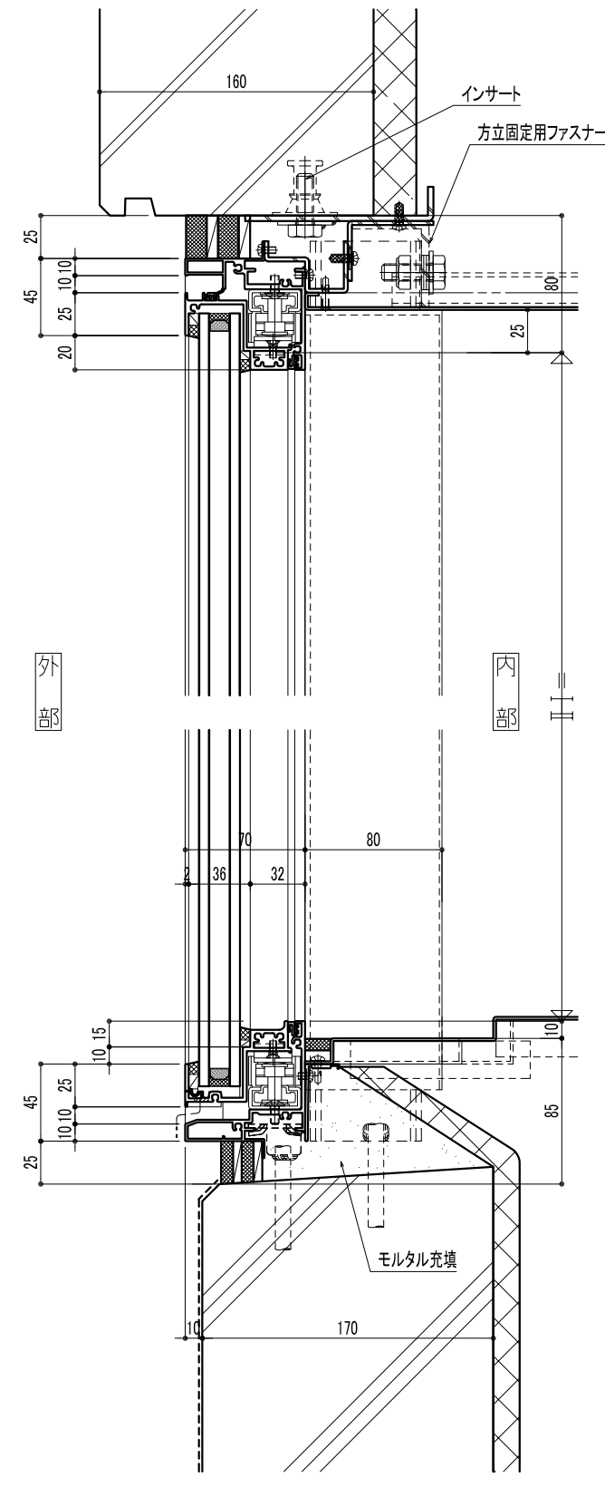
たてすべり出し窓部
