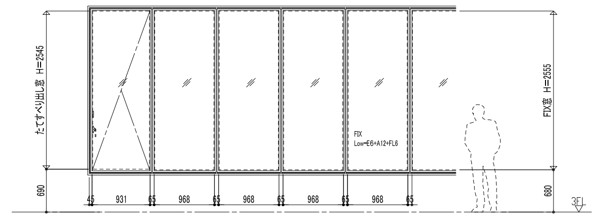
外観図 S=1/60
